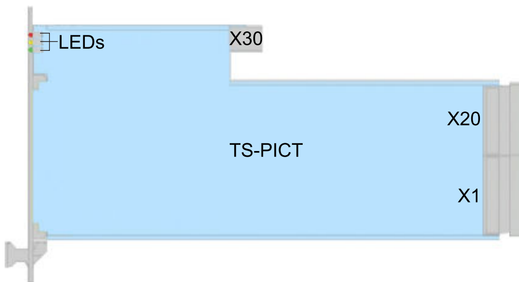
Bild 4-1: Anordnung der Steckverbinder am Modul R&S TS-PICT
