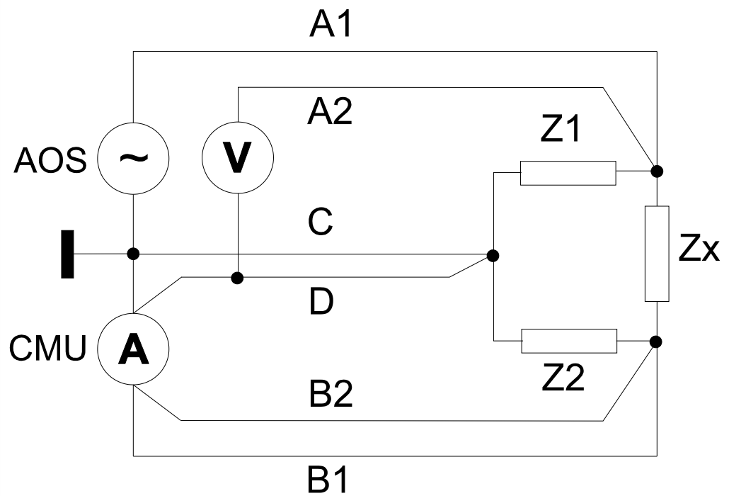
Bild 1-2: Verschaltung bei einer geguarterten Impedanzmessung (6- Draht)
