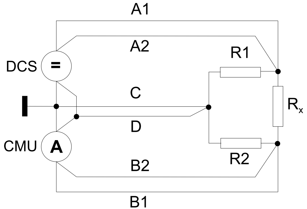
Bild 1-1: Verschaltung bei einer geguarterten Widerstandsmessung (6- Draht)
