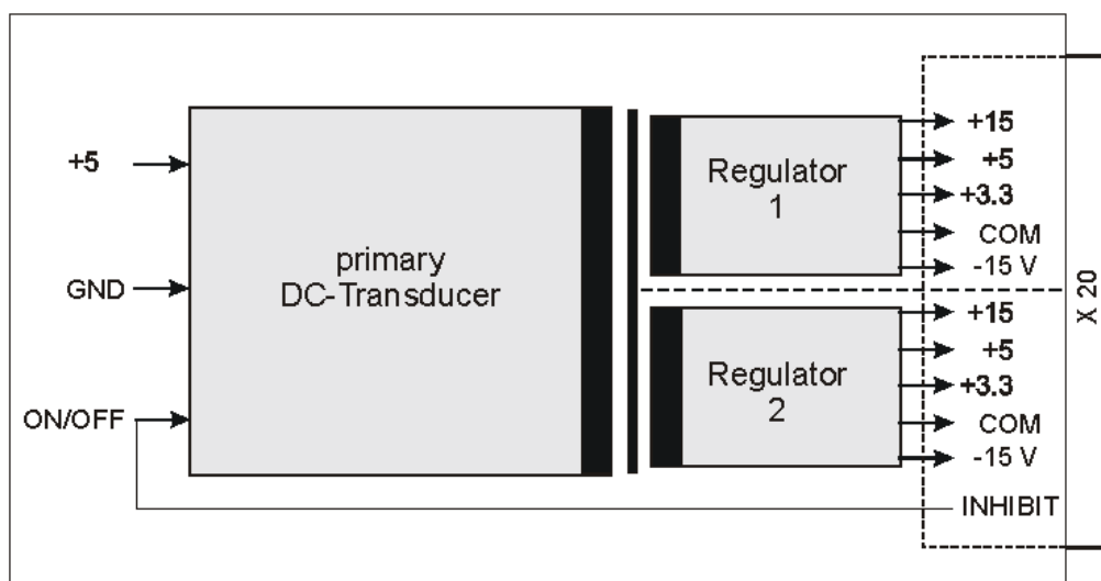
Bild 5-1: Blockschaltbild R&S TS-PDC
