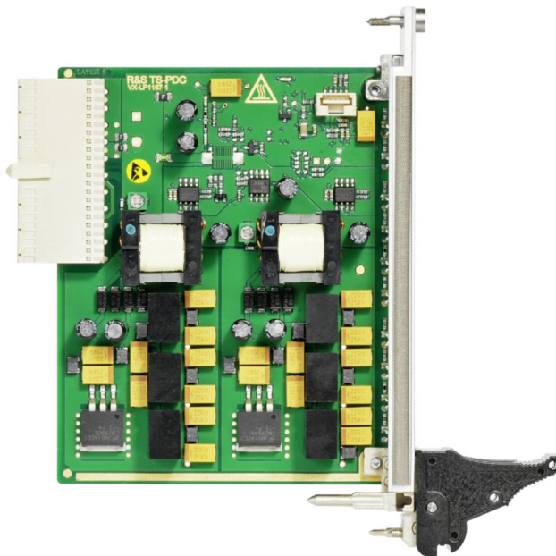
Bild 2-2: Ansicht des Rear-I/O Moduls R&S TS-PDC
