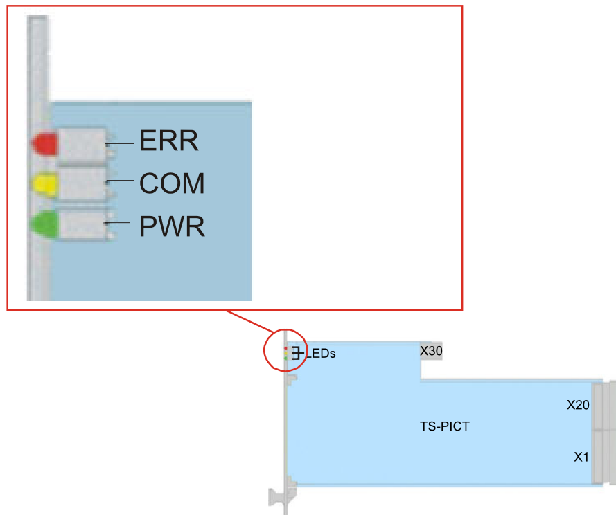
Bild 4-2: Anordnung der LEDs am Modul R&S TS-PICT
